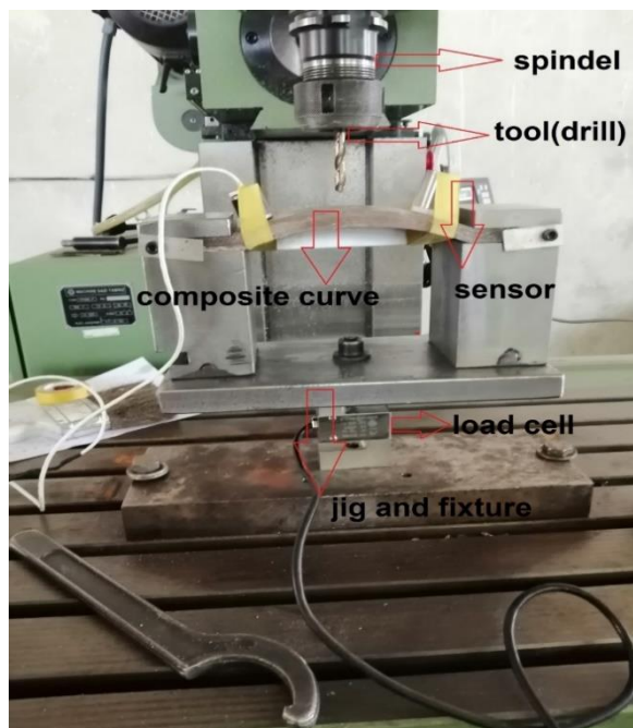
شکل ۷- مجموعه کامل آزمایش سوراخ کاری
