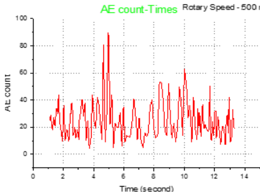
شکل ۱۱- سیگنال دریافتی نشر آوایی برحسب کانت
