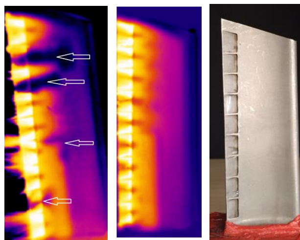
شکل ۴- نتیجه آزمایش دمانگاری برای نمونه پره شماره ۱ با و بدون انسداد کانالها
