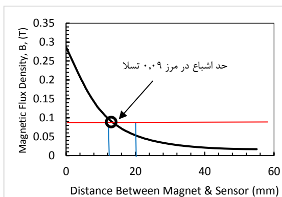
شکل ۳- تعیین فاصله بهینه برای قرارگیری آهنربا نسبت به حسگر
