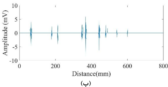
شکل ۵- حذف نویز سیگنال تجزیه شده در سطح d1 به روش حد آستانه، الف) سیگنال خام ب) سیگنال پردازش شده
