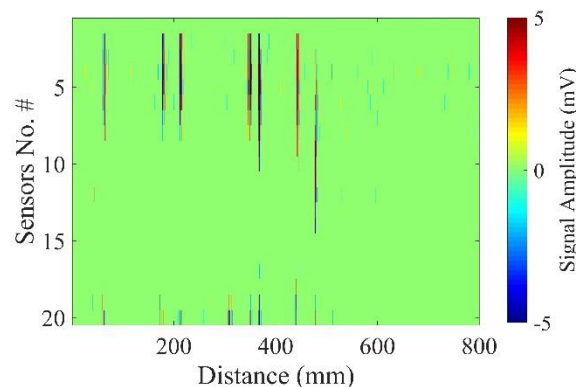
شکل ۶- تصویر حاصله از سیگنال های سطح d1 بعد از حذف نویز
