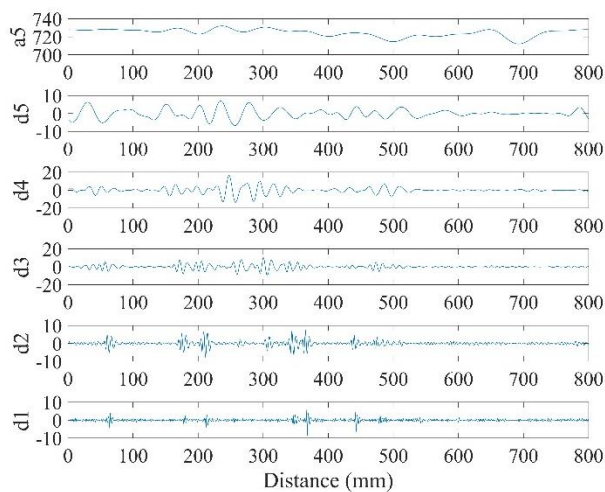
شکل ۴- تجزیه سیگنال به روش موجک در سطح ۵
