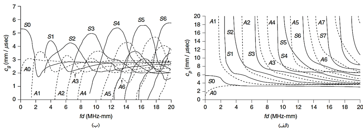
شکل ۱- نمودار دیسپرز آلومینیوم. (الف) سرعت فاز، (ب) سرعت گروه [۱]
