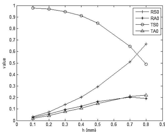
شکل ۵- نمودار ضرایب عبور و بازتاب برحسب مقادیر مختلف h در ورق با تغییر ضخامت مشابه سایش
