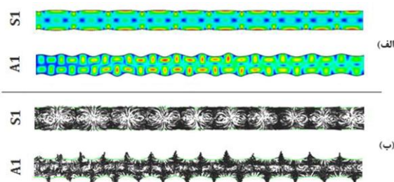
شکل ۶- الف) توزیع تنش معادل فون-مایز و ب) توزیع جابجایی برآیند در مدهای S1 و A1 در فرکانس-ضخامت 4 MHz.mm
