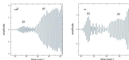
شکل ۷- جابجایی نقطه‌ای بر روی سطح ورق در مدهای A1 و S1، الف: مولفه جابجایی در-صفحه ب: مولفه جابجایی خارج-از-صفحه در فاصله 100 mm از لبه ورق
