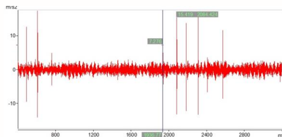
شکل ۸- موج زمانی جهت به دست آوردن فرکانس خرابی اجسام دورانی
