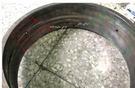
شکل ۹- وضعیت حلقه خارجی یاتاقان پس از تعویض
