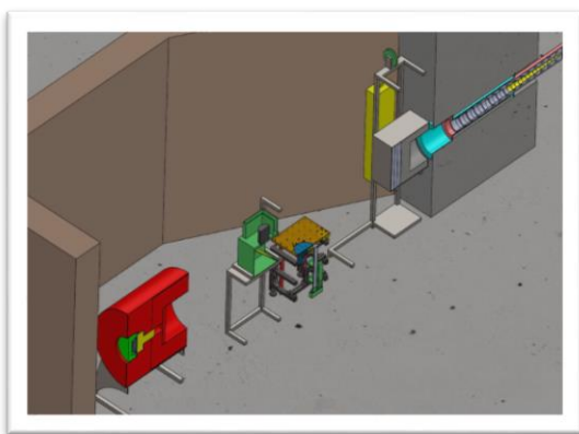
شکل ۵- اتاق رادیوگرافی نصب شده در باریکه E و نمائی برش خورده از کالیما تور، شاتر، میز رادیوگرافی، متوقف کننده بیم و دیوارهای بتونی
