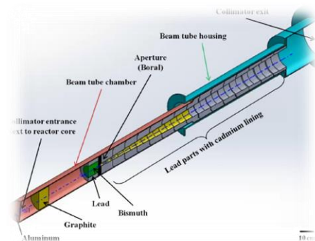
شکل ۴- نمائی از راکتور تحقیقاتی تهران، بیم تیوب‌های آن و بیم تیوب مورد استفاده E در این تحقیق به همراه نمائی از کالیما تور نوترونی طراحی شده
