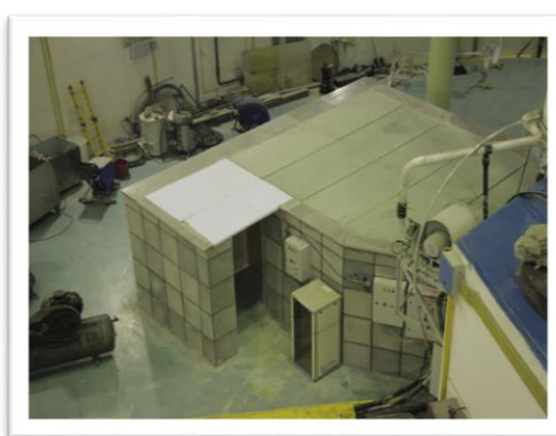
شکل ۵- اتاق رادیوگرافی نصب شده در باریکه E و نمائی برش خورده از کالیما تور، شاتر، میز رادیوگرافی، متوقف کننده بیم و دیوارهای بتونی
