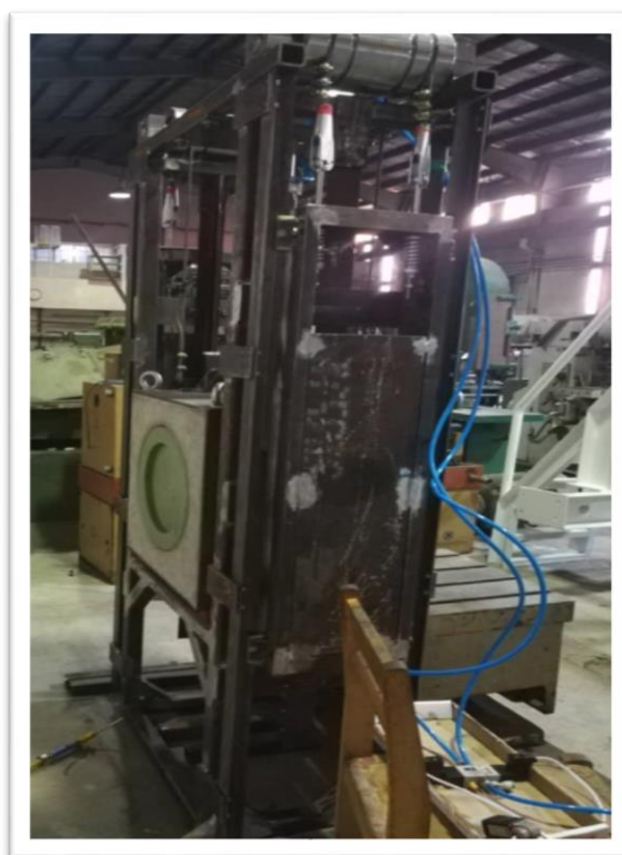
شکل ۶ - نمائی از شاتر بیم نوترونی: طراحی، ساخت و نصب
