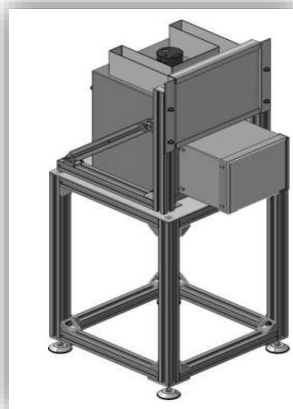
شکل ۹ - سیستم تصویربرداری دیجیتال نوترونی با زمان حقیقی و روش پریسکوپ برای جلوگیری از آسیب به دوربین به همراه نمای طراحی محفظه پریسکوپ و دوربین
