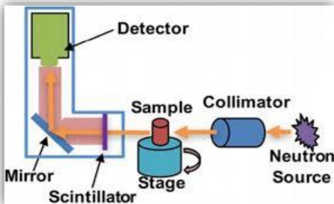
شکل ۹ - سیستم تصویربرداری دیجیتال نوترونی با زمان حقیقی و روش پریسکوپ برای جلوگیری از آسیب به دوربین به همراه نمای طراحی محفظه پریسکوپ و دوربین
