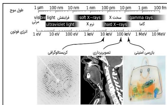
شکل ۱- محدوده طول موج و انرژی فوتون
