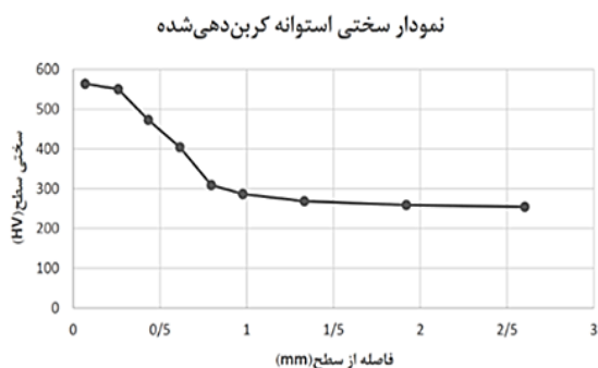
شکل (۴): نمودار سختی واقعی قطعه سخت‌کاری‌شده.
