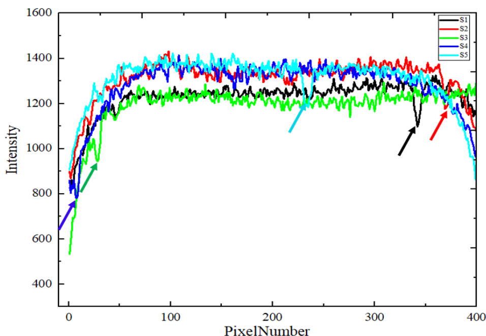
شکل ۱۰) مقایسه تغییرات شدت ثبت شده در آشکارساز به ازای خط افقی در پنج نمونه در راستای خط گذرنده A به تفکیک افشانه‌ها (بردارها نشان دهنده افت در شدت ثبت شده به سبب حضور خط جوش روی بدنه)
