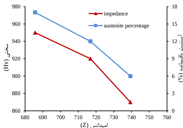
شکل (۸) ارتباط میان میزان آستنیت باقیمانده و جریان گردابی (امپدانس) برای سه نمونه ۴۰۲ و ۶.
