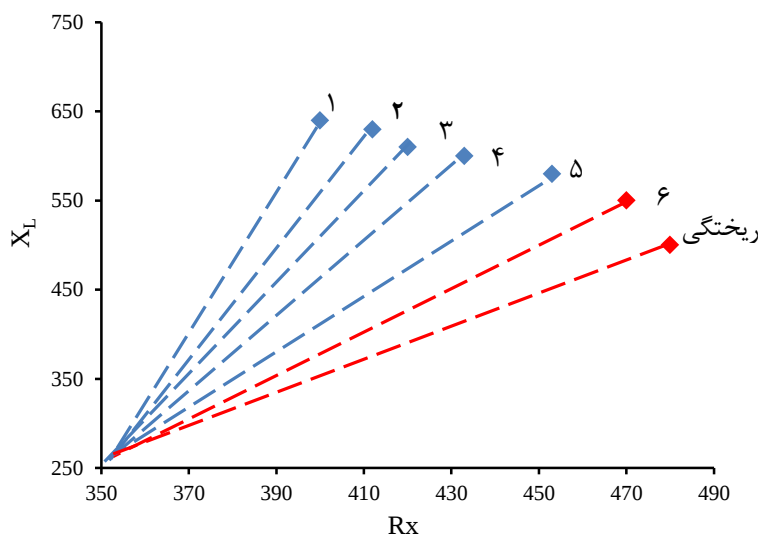
شکل (۶) تاثیر ریزساختار نمونه‌ها بر روی نحوه قرارگرفتن نقاط در صفحه امپدانی.
