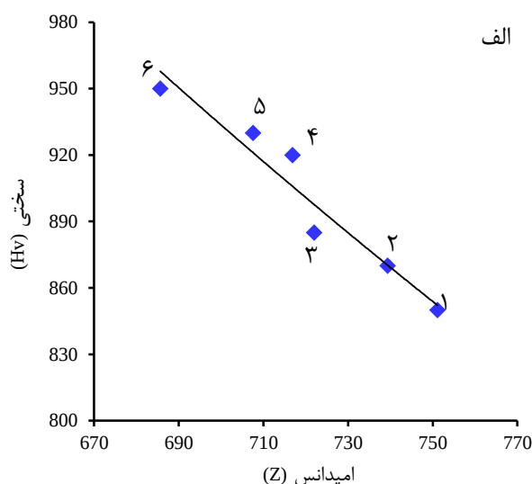
شکل (۷) ارتباط میان شاخص‌های جریان گردابی با سختی در شرایط مختلف عملیات حرارتی الف: شاخص Z ب: XL.
