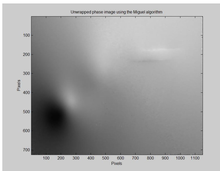
شکل ۷. تعیین عیوب زیرسطحی ورقه‌ی پلکسی شامل حفره‌ای به قطر ۱۲ mm و ترکی به عرض ۰/۵ میلی‌متر و طول ۲ سانتی‌متر
