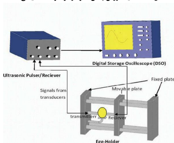
شکل ۵- تعیین تازگی تخم مرغ با فراصوت [۴۸]
